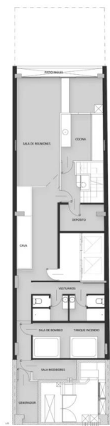
PIANTA SÓTANO
