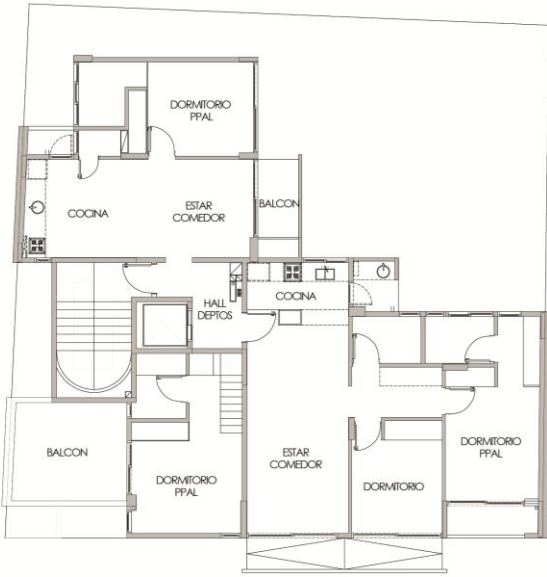
SEXTO PISO
