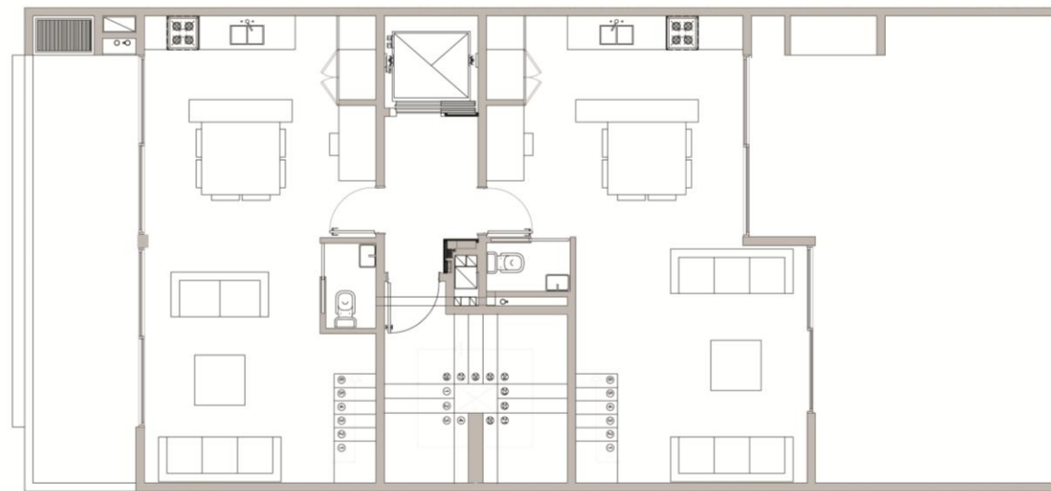
PLANTA TIPO 1
